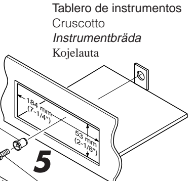
Perno de montaje Bullone di montaggio Monteringsbult Kiinnityspultti
